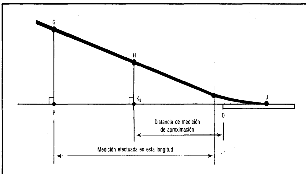
Figura 2-9. Perfil típico de aproximación
