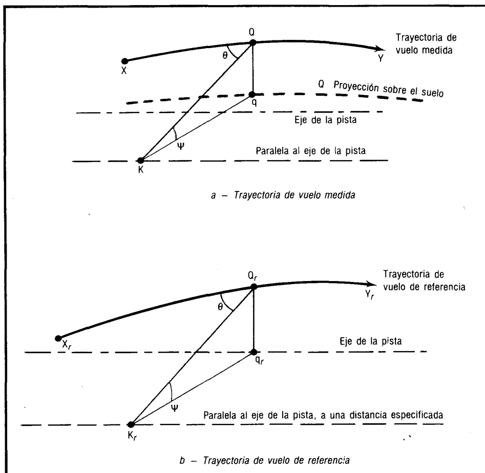
Figura 2-11. Medición lateral — determinación de la estación de referencia
