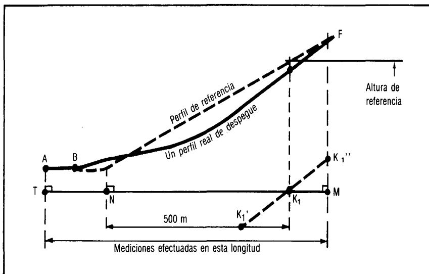
Figura 2-4. Perfiles típicos de ensayo y de referencia
