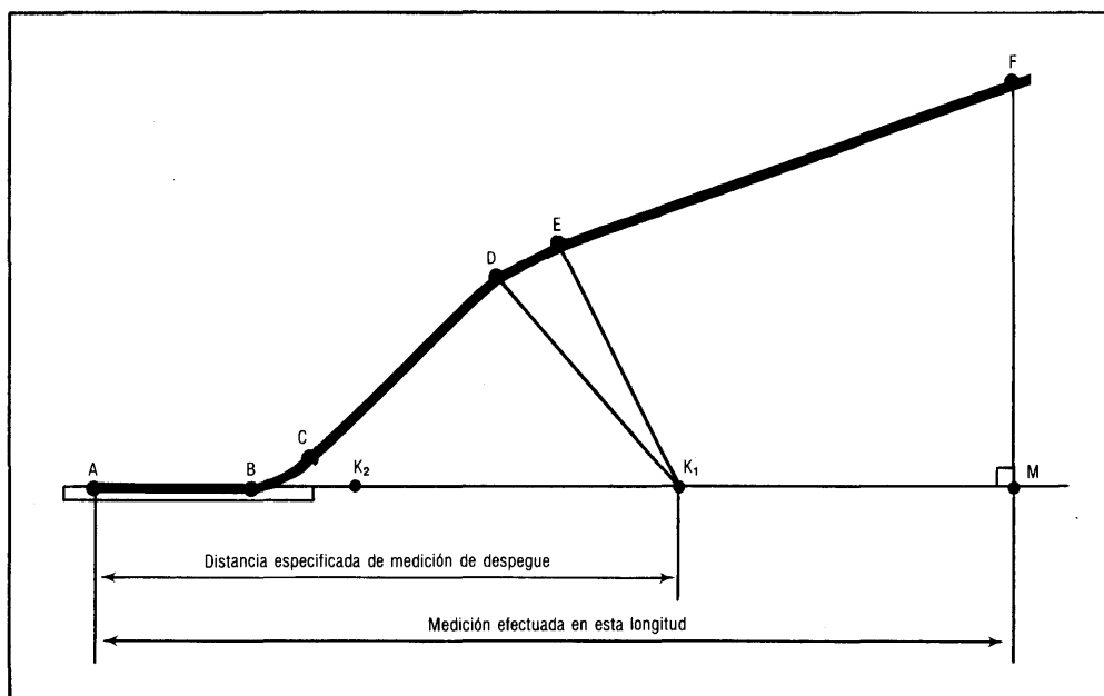
Figura 2-8. Perfil típico de despegue
