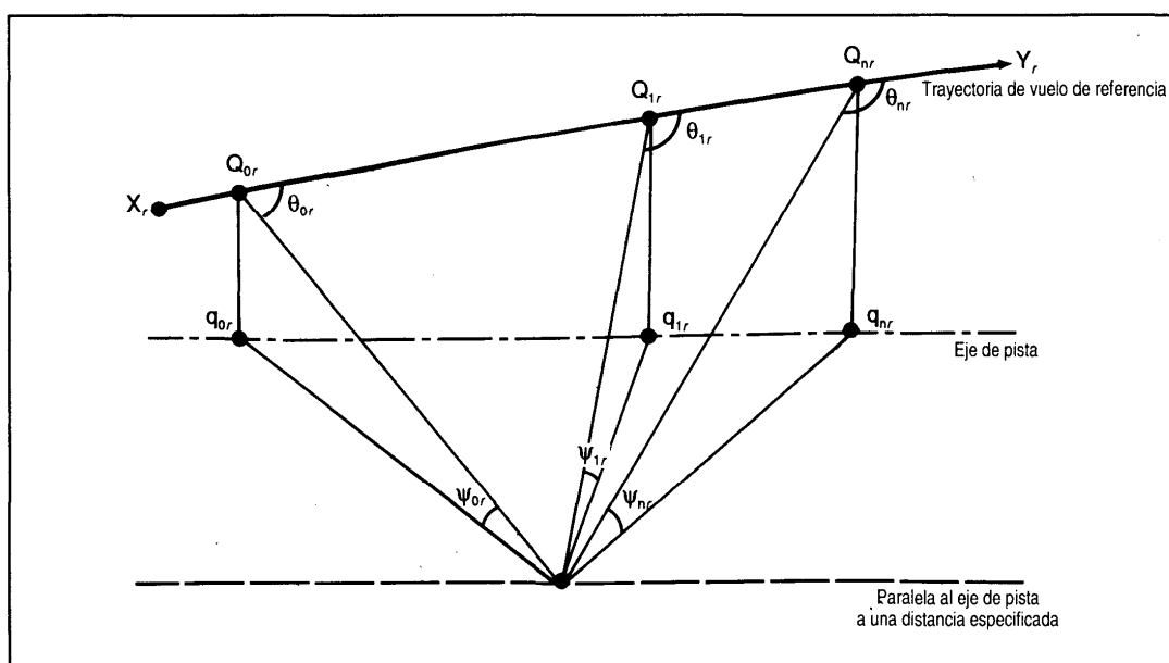
Figura 2-15 b). Trayectoria de vuelo de referencia
