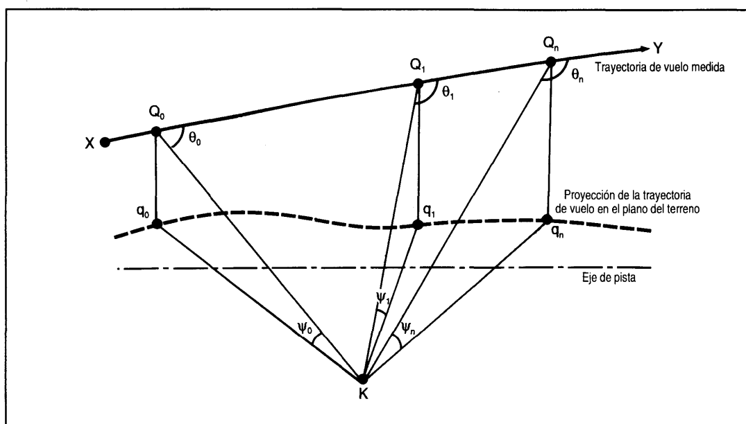
Figura 2-15 a). Trayectoria de vuelo medida
